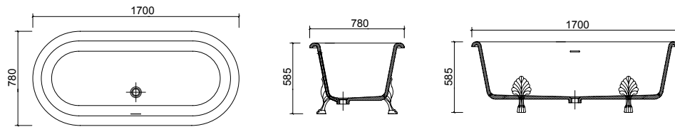
BT030127 1700 x 780 x 585mm
