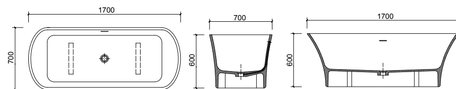
BT030104 1700 x 700 x 600mm
