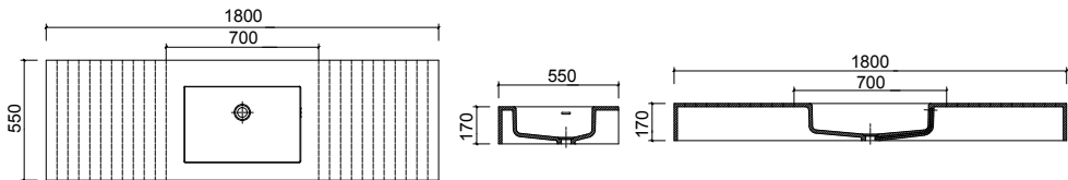
BA060056 700~1800 x 550 x 170mm
