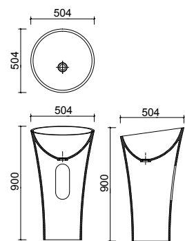
BA050017 504 x 504 x 900mm
