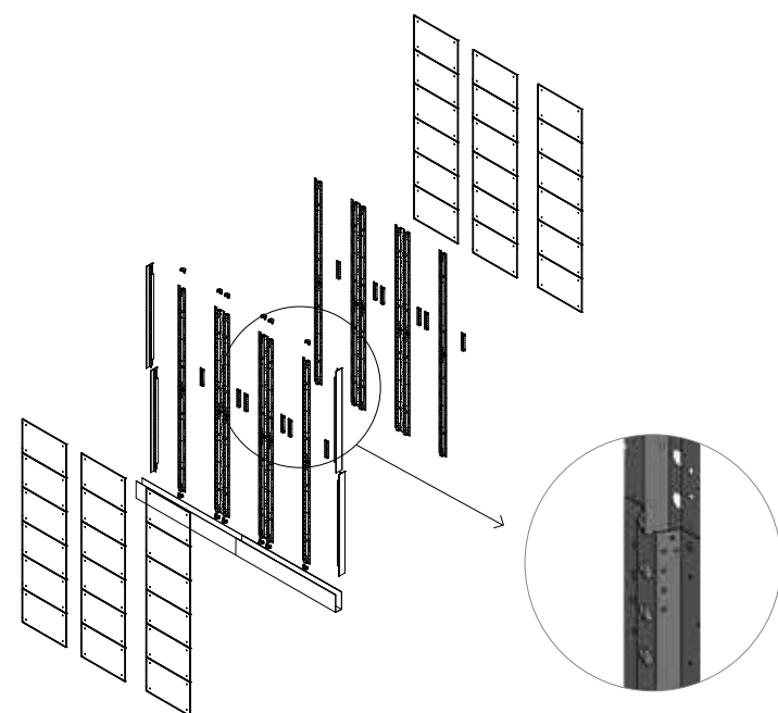
Layout - Schema di posa
