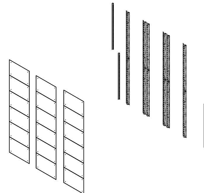
Layout - Schema di posa
